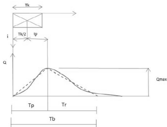
Slika 1.b: Jedinični hidrogram
